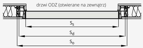
DRZWI OTWIERANE NA ZEWNĄTRZ ODZ
