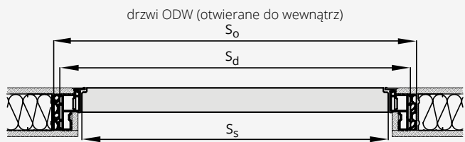
DRZWI OTWIERANE DO WEWNĄTRZ ODW
