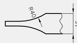
profil płyciny MDF 16 mm (Piano 1, 2, 5, 6)
