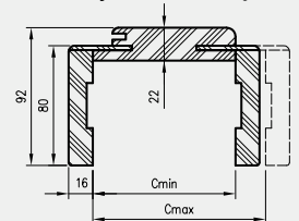
Przekrój OR/ORC z ką. T80
