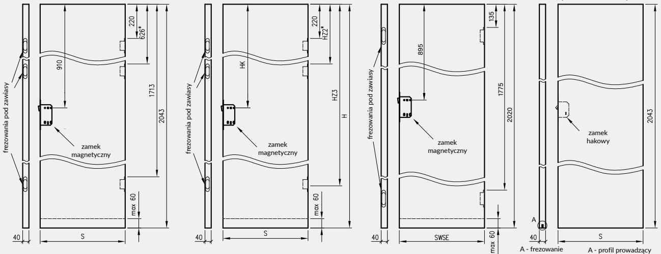
Skrzydła przesuwne do: - kaset ościeżnicowych PA - systemów SPAZIO CD - systemów naściennych
